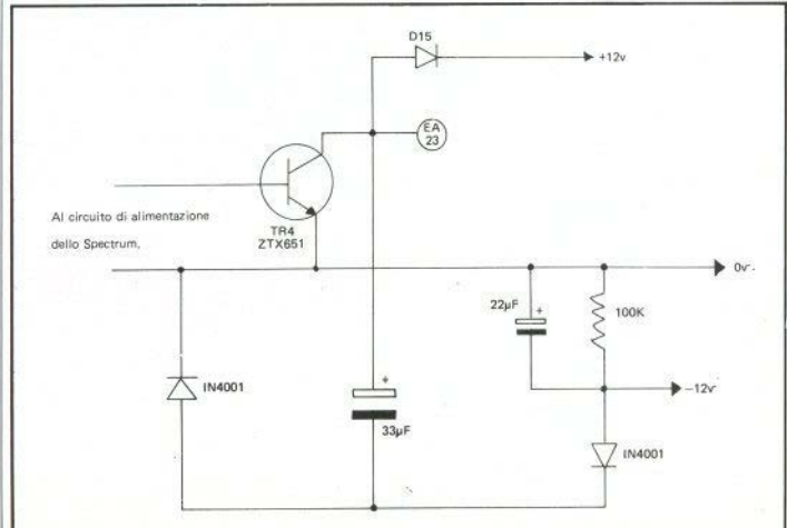
Fig. 5. Circuito supplementare per alimentazione -12V
